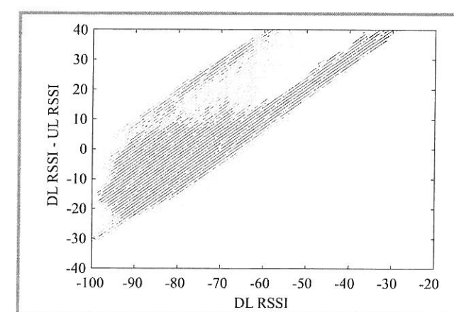
Fig. 10. DL RSSI vs. DL RSSI - UL RSSI.
