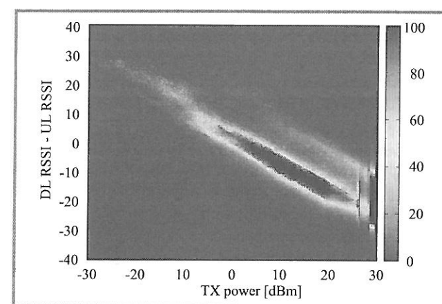
Fig. 11. CPE TX power vs. DL RSSI - UL RSSI.
